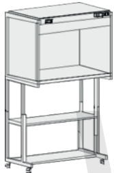
C28-A Modelo: CMB-2028/FS
